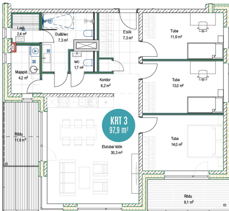
KORTERI PLAAN
