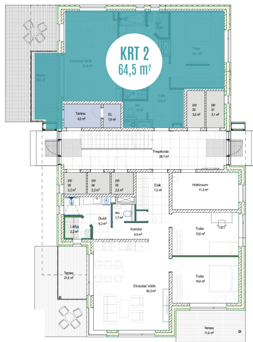
KORRUSE PLAAN
